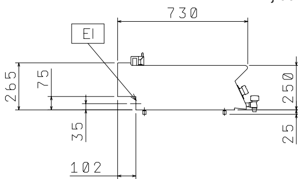
Zij aanzicht
